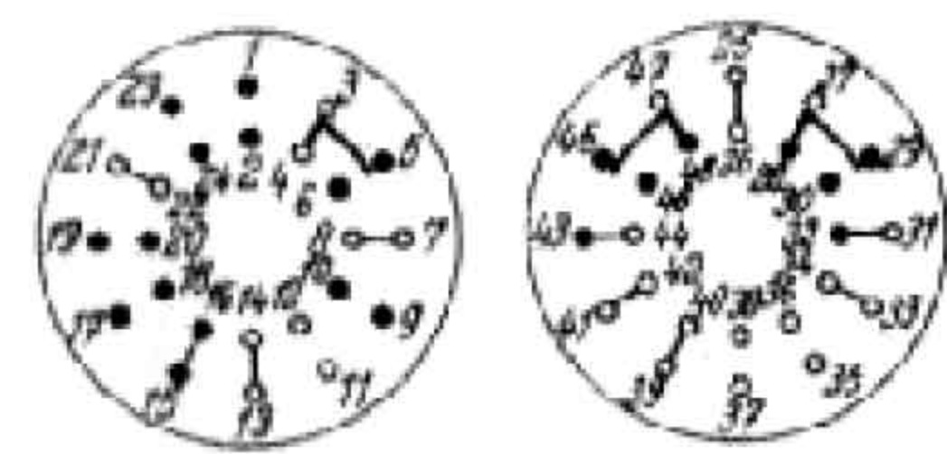
Vorkreis u. Oszillator Gezeichnete Stellung - UKW
